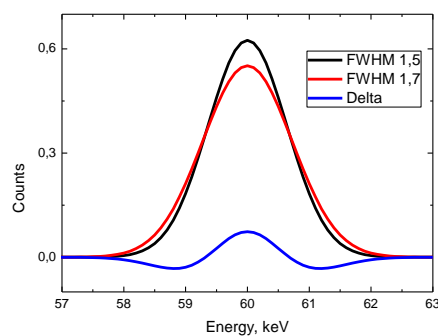
Рис. 6 б. Расчетные пики излучения с энергиями в максимуме 60 кэВ. Ширины на полувысоте FWHM составляют 1,7 и 1,5 кэВ. Delta – результат вычитания спектров
