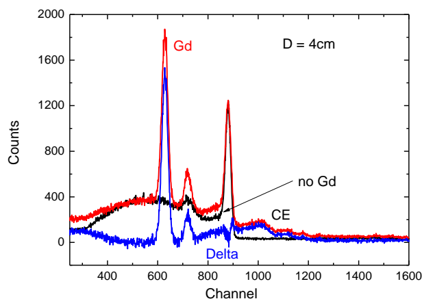
Рис. 10. Экспериментальные спектры, измеренные двумя детектирующими модулями Si, 5 \times 5 мм 2 с гадолиниевым конвертором и без. Delta – разница спектров излучения. D = 4 см
