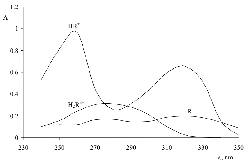
Рис. 4. Електронні спектри поглинання R , HR^+ , H_2R^{2+} форм 3-(трифлуороацетил)імідазо[1,2-а]піримідину у розчині ЦДАПС ( 1 \times 10^{-2} М).
