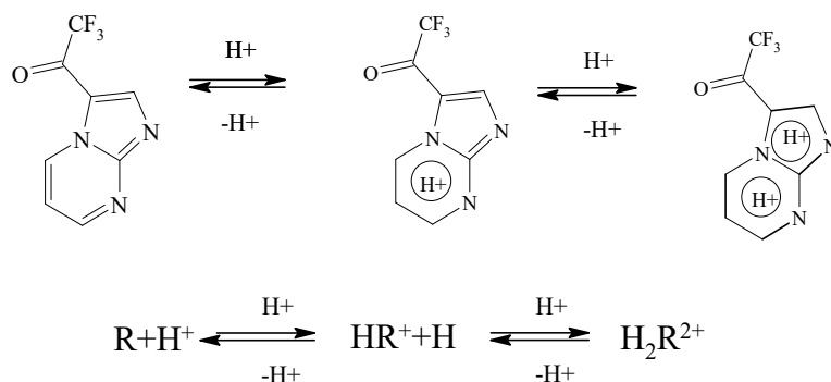
Схема 1. Протолітичні рівноваги 3-(трифлуороацетил)-імідазо[1,2-а]піримідину у водних розчинах.
