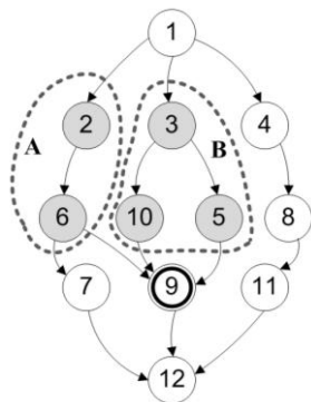
Рис. 5. Принцип восстановления данных (backtracking)
