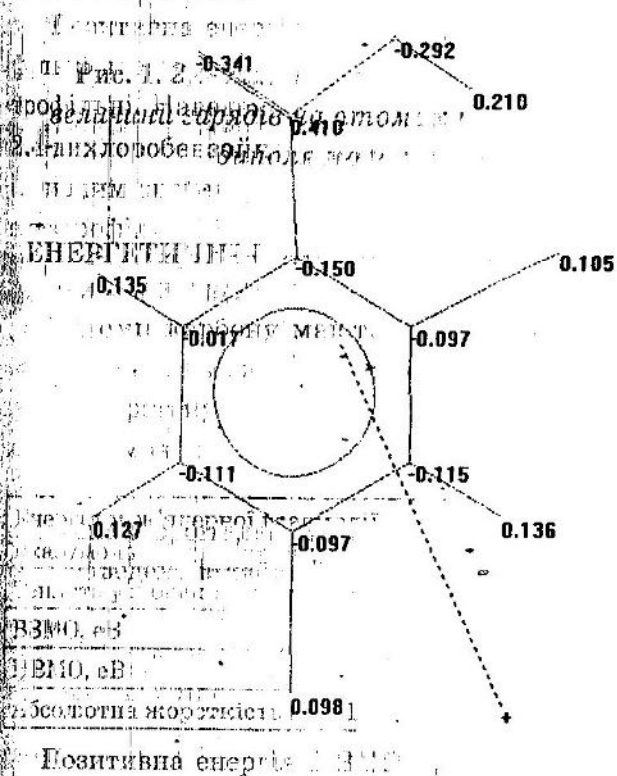
Рис. 1. 2,4-дихлоробензойна кислота - величини зарядів на атомах та напрямок диполя в молекулі.
