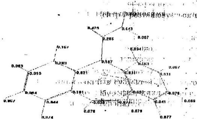
Рис. 3. Величини зарядів на атомах та напрямок диполя молекули карбамазепіну.
