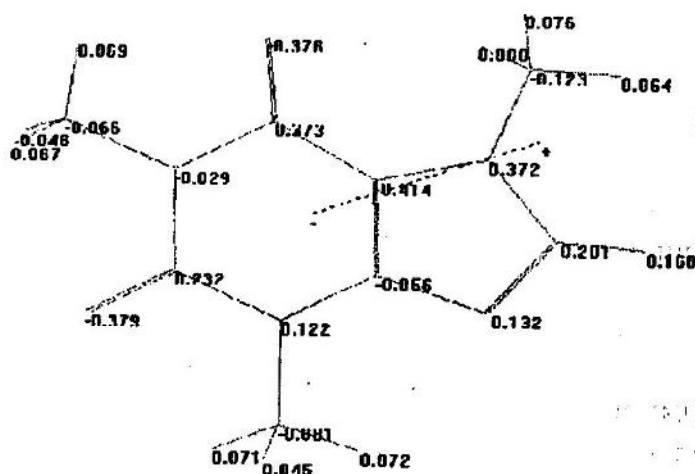
Рис. 2. Кофеїн - заряди на атомах та напрямок диполя на його молекулі.
