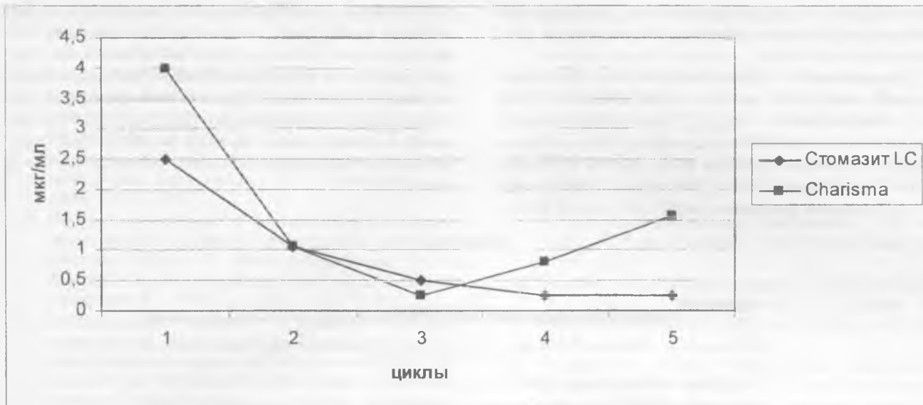
Рис. 1. Диффузия ионов фтора в модельную среду из ФКМ
