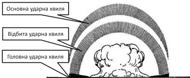
Схема утворення ударних хвиль при повітряному вибуху
