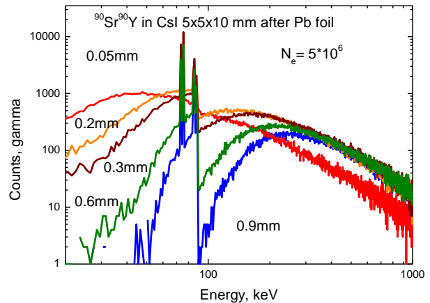
Рис. 7. Результаты расчета энергетических спектров гамма квантов, возбуждаемых ^{90}\text{Sr}+^{90}\text{Y} в детекторе CsI(Tl) размером 5 \times 5 \times 10 мм для Pb фольг различных толщин, мм. Fig. 7. The results of calculation of energy spectra of gamma rays excited by ^{90}\text{Sr}+^{90}\text{Y} in the CsI(Tl) detector of size 5 \times 5 \times 10 mm for Pb foils of different thicknesses, mm.
