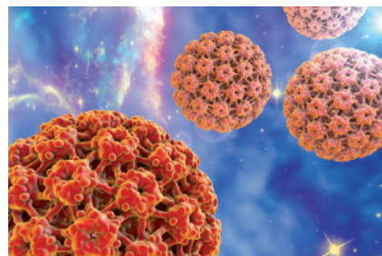
Папилломавирус человека
