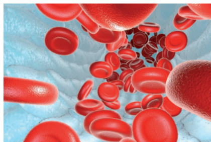
Эритроциты
