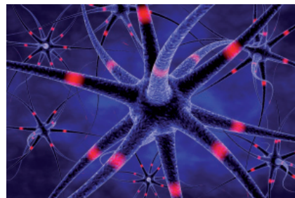
Нейроны
